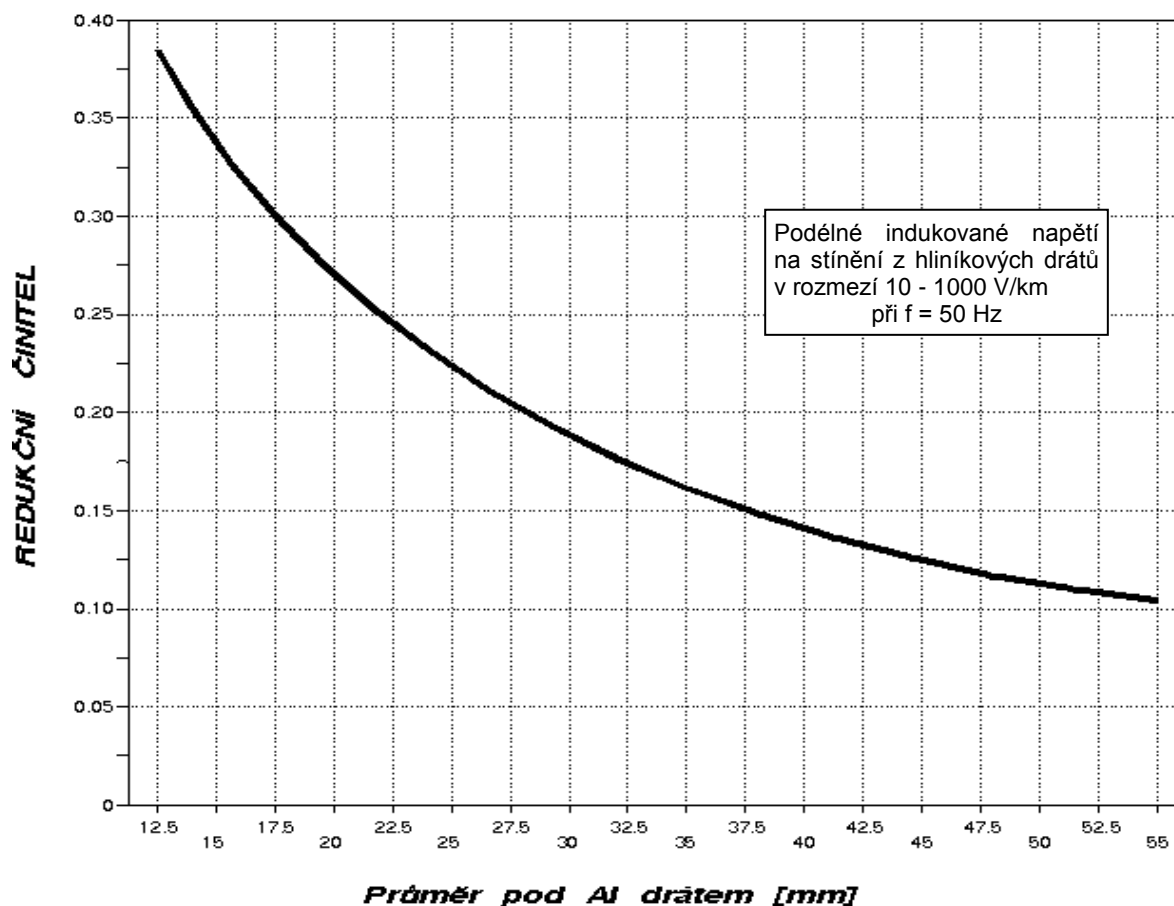
graf č. 1 Redukční činitel kabelů v provedení AJ-HHAH (...AL) a AJ-HHAH-J (...AL)
